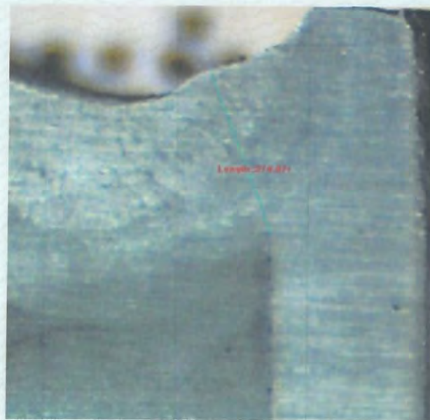
شکل 30. تصویر ماکروسکوپی از مقطع عرضی آماده سازی شده. (مقطع 30) محلول ظاهر کننده: نایتال ده درصد
