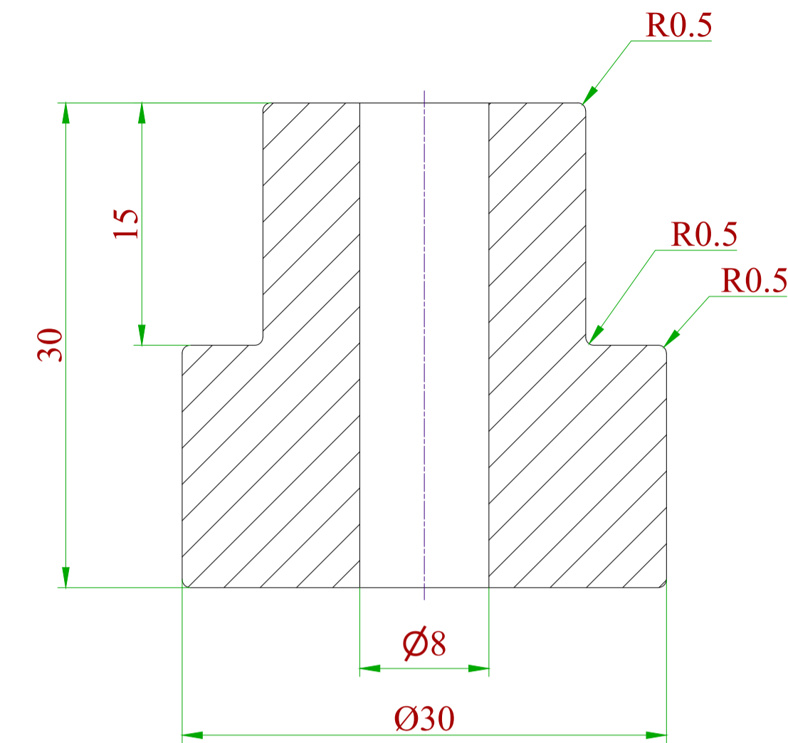
Pos. 11 : Bush View Scale : ( 2 : 1 )
