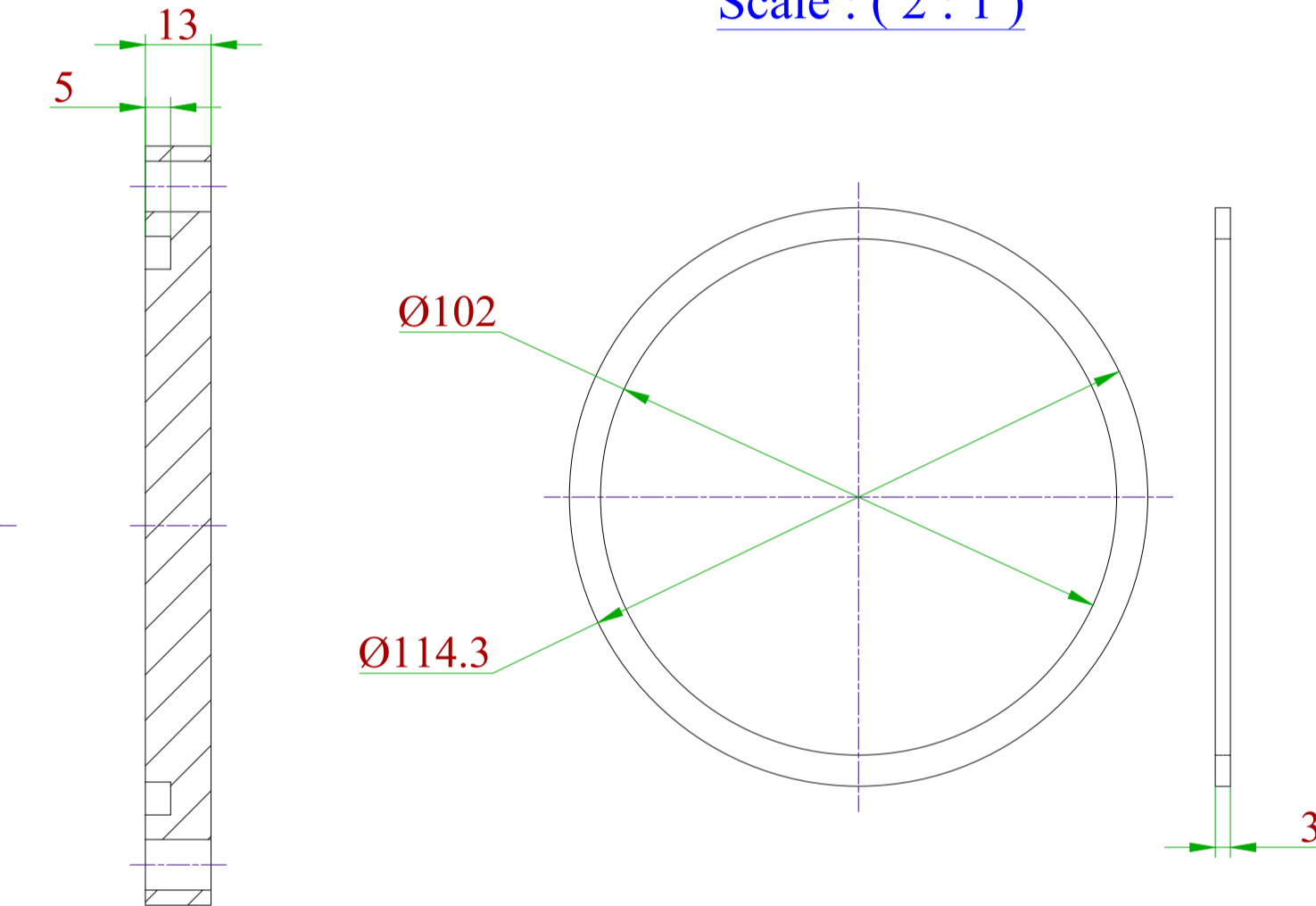
Pos. 03 : Seal Ring View Scale : ( 1 : 2)
